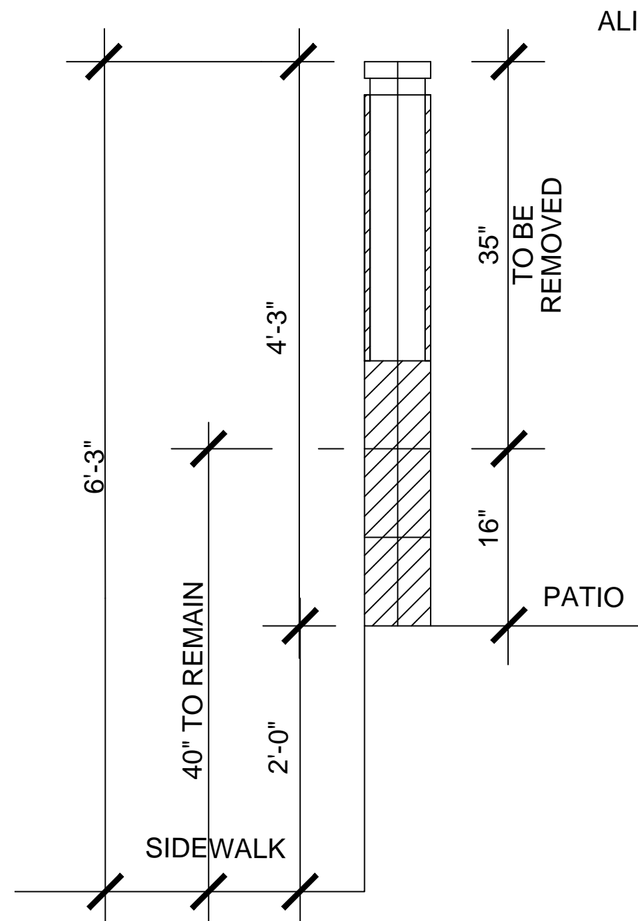
EXISTING ELEVATION A - A SCALE: 1" = 1'-0"
